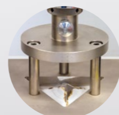
Átütőmunka (LPET) DIN 53142-2
