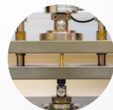
Élőnyomó szilárdság (ECT) ISO 3037
