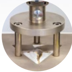
Durchstoßprüfung (LPET) DIN 53142-2
