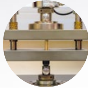
Kantenstauchwiderstand (ECT) ISO 3037
